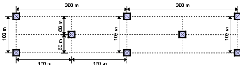
Figura 1. Disposición de dos grupos básicos de bloque disuasivos (X). El lado mayor se sitúa paralelo a la costa.
