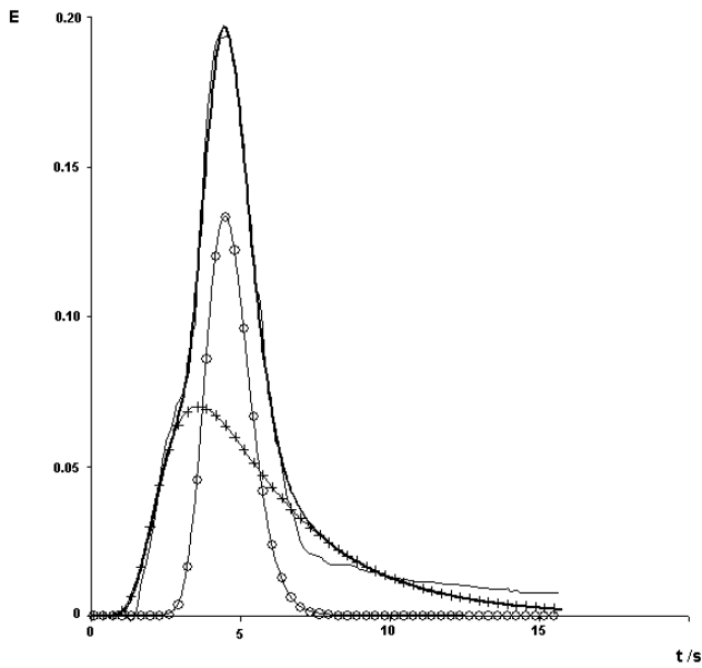
Fig. 3. Superposición de las curvas experimental y calculada para un caudal volumétrico de 105 l/h; + Camino 1; o Camino 2; - Experimental,
