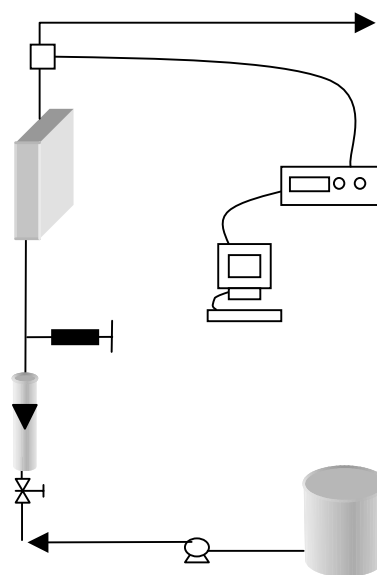
Diagrama del montaje experimental
