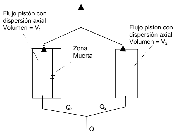
Fig. 1. Esquema del modelo para la caracterización de flujo
