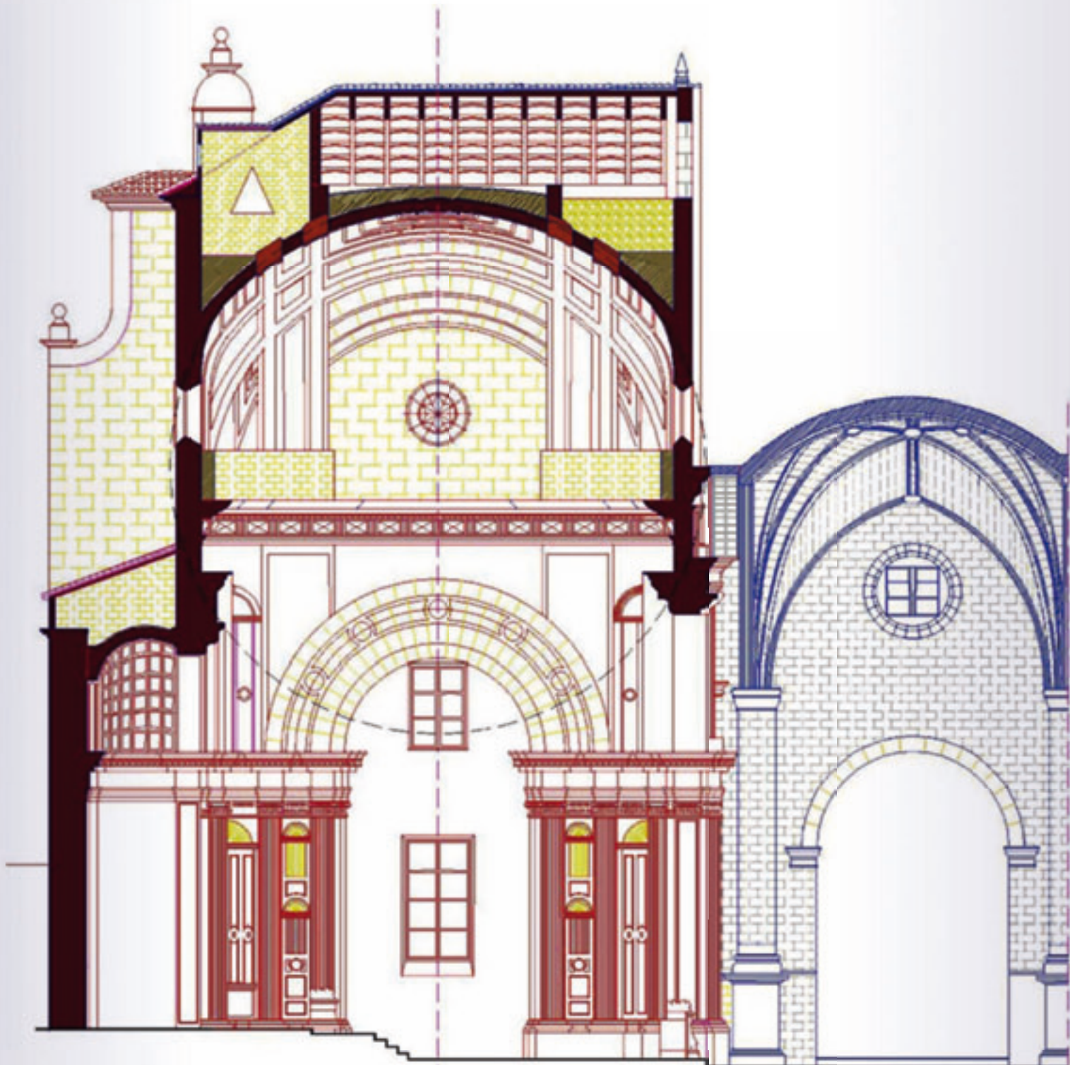
Sección longitudinal a eje de cabecera
