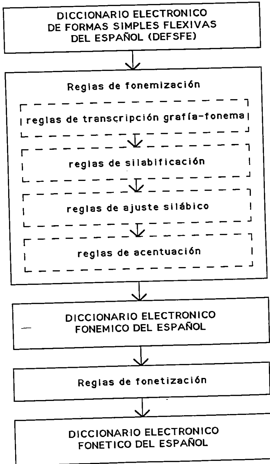
Figura 1. Estructura del Diccionario Electrónico Fonético del Español (DEFE).
