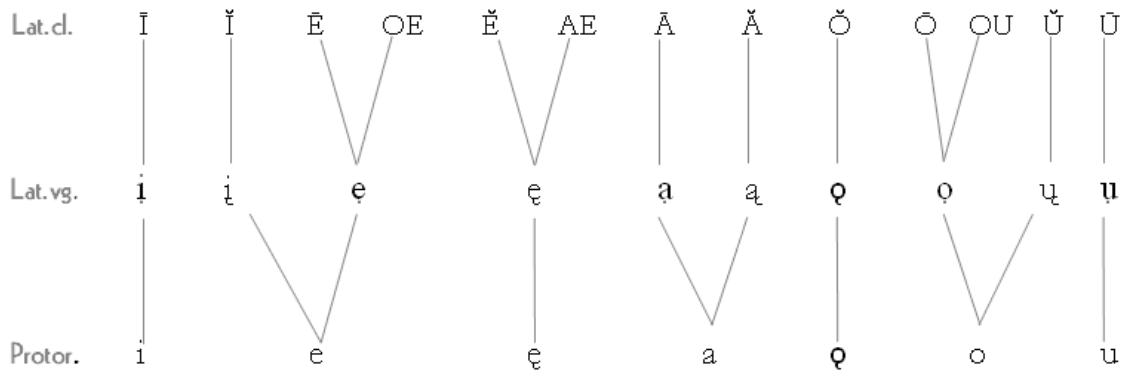
Fig. 3: Evolución del sistema vocálico desde el lat. cl. al protorromance
