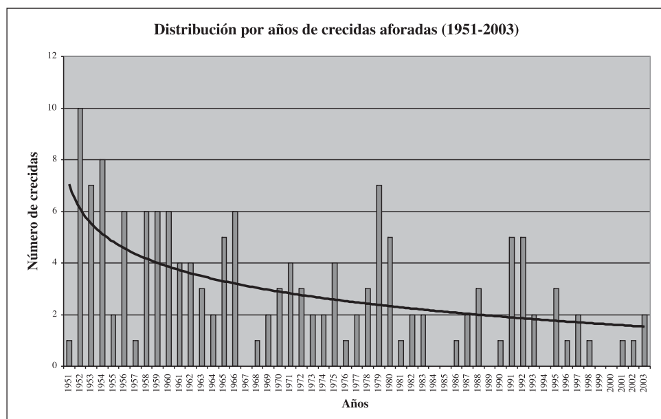
FIGURA 4. Distribución de crecidas por años (1951-2003). Elaboración propia.
