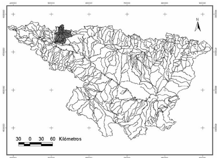
FIGURA 1. La cuenca del río Zadorra en la cuenca del río Ebro. (Fuente: Confederación Hidrográfica del Ebro. Elaboración propia).
