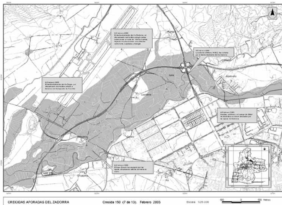
FIGURA 5. Crecida de febrero de 2003 en el entorno de la ciudad de Vitoria-Gasteiz. (Fuente: Trabajo de campo. Elaboración propia).
