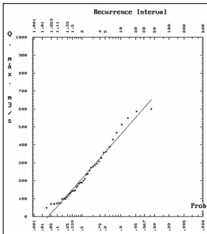
FIGURA 6. Ajuste de Gumbel. (Fuente: RANKPLOT. Elaboración propia).
