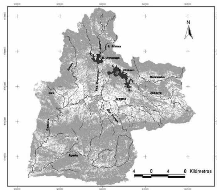
FIGURA 2. La cuenca del río Zadorra. (Fuente: Gobierno Vasco. Elaboración propia).
