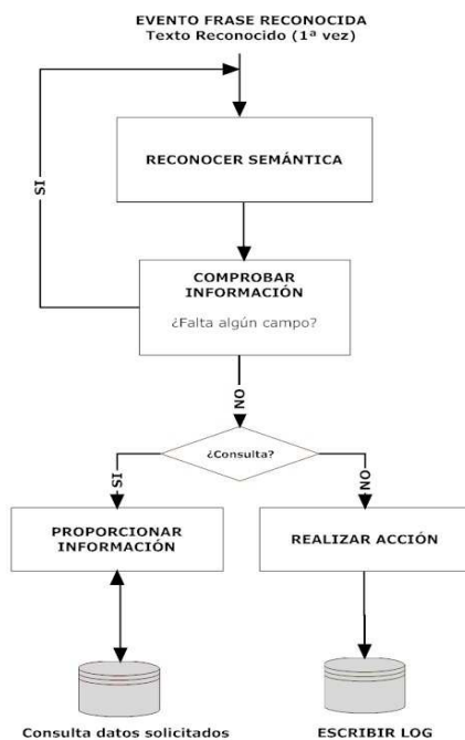
Figura1. Proceso seguido por el gestor del diálogo
