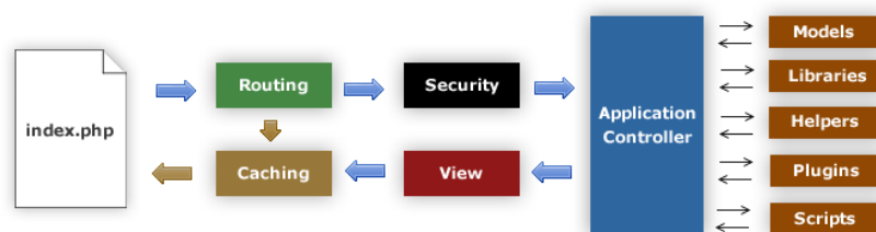
Figura 7: Flujo de ejecución de CodeIgniter
