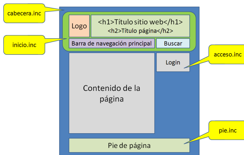
Figura 6: Plantilla de una página web
