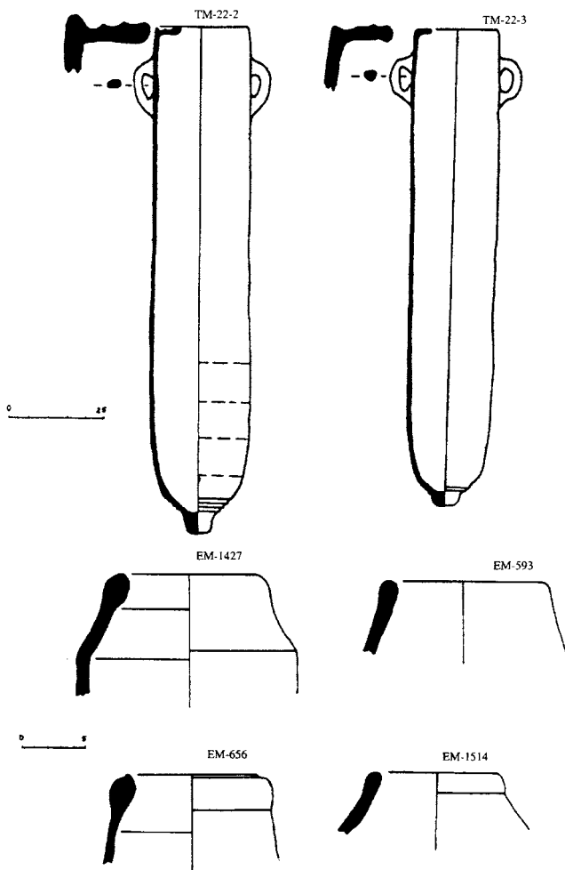
Lámina nº 3: Mañá D (TM-22-2, TM-22-3). Mañá Pascual A4 (EM-1427, EM-593, EM-656, EM-1514).
