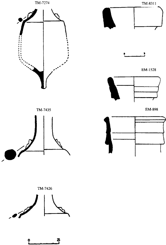
Lámina nº 18: Lamboglia 2 y variantes apulas.
