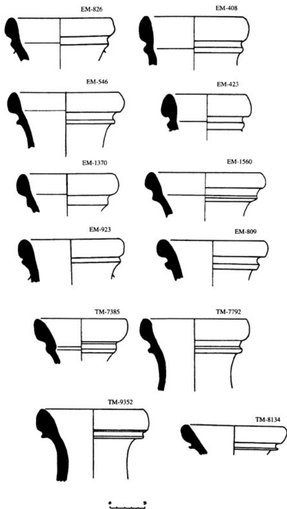
Lámina nº 19: Lomba do Canho 67.
