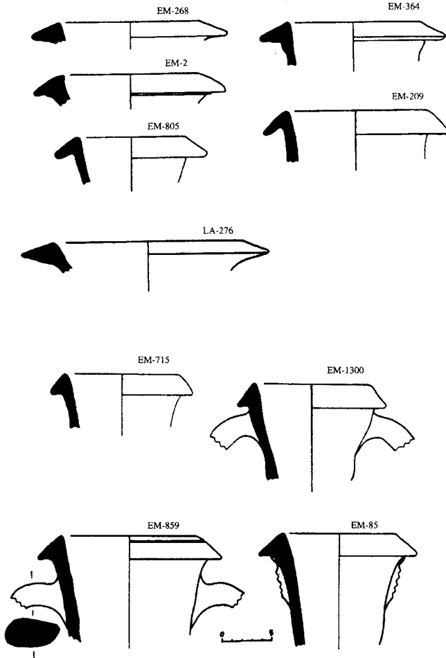
Láminanº 12: Grecoitálica antigua: EM-268, EM-2, EM-805, LA-276, EM-364, EM-209. Grecoitálica clásica: EM-603, EM-715, EM-859, EM-285, EM-1300, EM-85.
