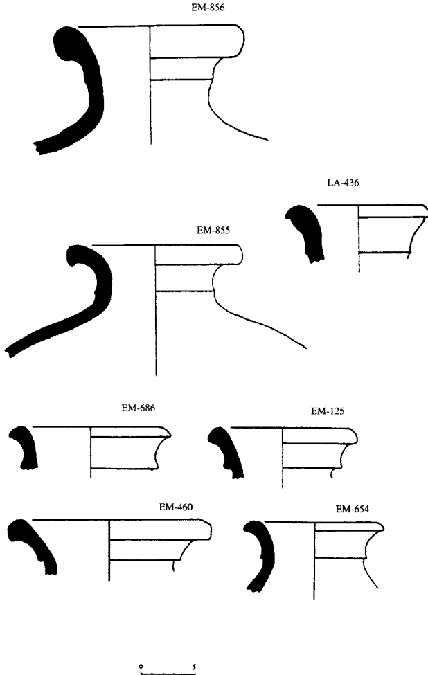
Lámina nº 4 Mañá C Grande (EM-856, EM-855) Mañá C Cartagena 1 (LA-436, EM-686, EM-125, EM-460, EM-654)
