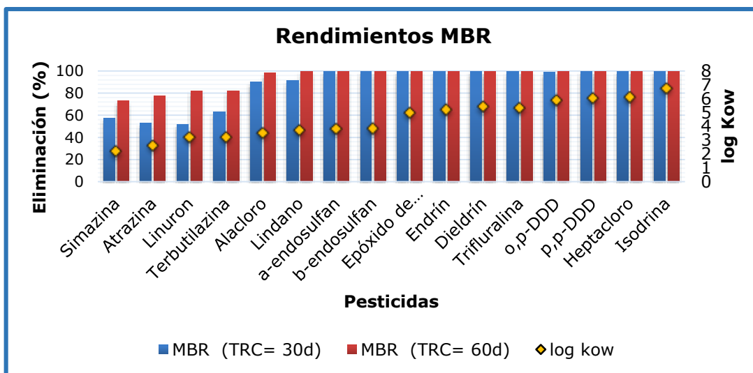
Figura 2. Eliminación media de los pesticidas.
