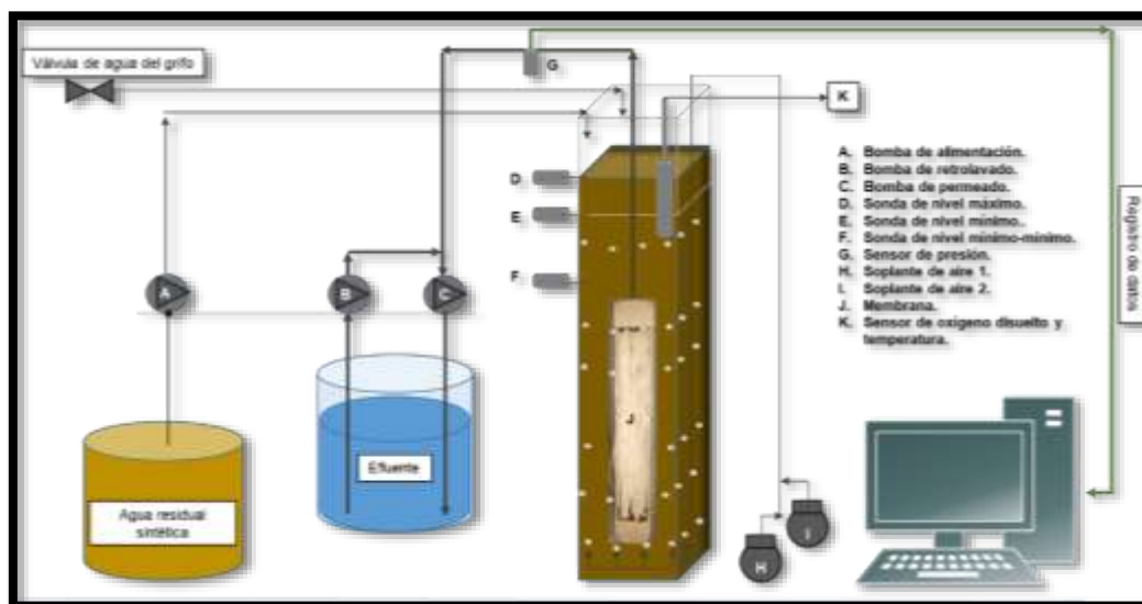
Figura 1. Esquema de la planta piloto.
