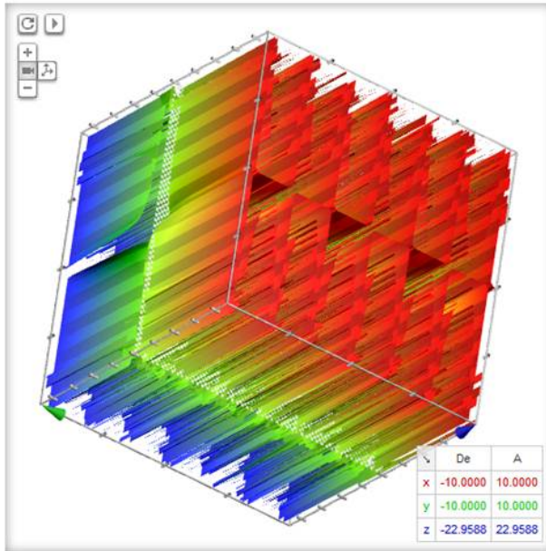
Gráfico de \cos(y)/\sin(x*\tan(y))-2
