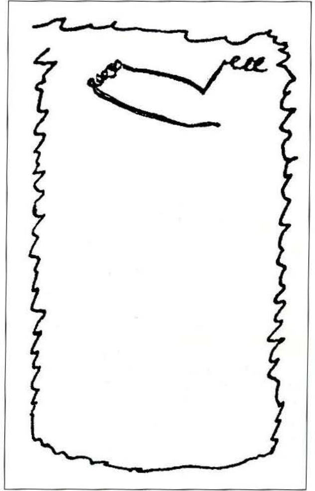
Fig. 2.- Planta de la sepultura y parte del ajuar (fibula), según Flores
