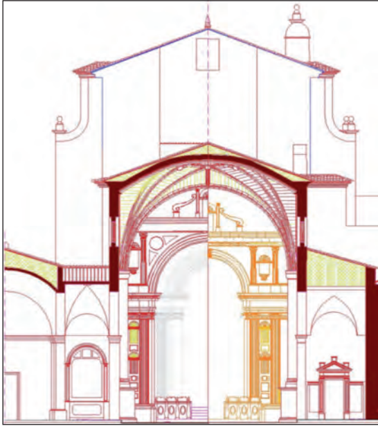
Fig. 5.- Iglesia de Santiago en Orihuela –Alicante-. Sección transversal desde la nave hacia la cabecera representando dos alternativas de solución del arco de triunfo de acceso a la misma. Dibujo inédito derivado de la tesis doctoral de LÓPEZ GONZÁLEZ, Antonio Luis, op. cit.
