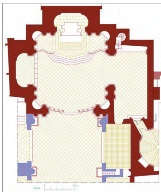
Fig. 4.- Iglesia de Santiago en Orihuela –Alicante–. Fragmento de la planta, conteniendo la Capilla Mayor y el último tramo de la nave gótica. Dibujo inédito derivado de la tesis doctoral de LÓPEZ GONZÁLEZ, Antonio Luis, op. cit.
