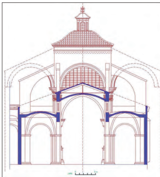
Fig. 2.- Iglesia de Santa María del Salvador de Chinchilla de Montearagón. Sección transversal proyectada hacia la cabecera renacentista; se propone una solución de posible reconstrucción de los arcos propios de una iglesia salón. Dibujo inédito derivado de la tesis doctoral de LÓPEZ GONZÁLEZ, Antonio Luis, op. cit.
