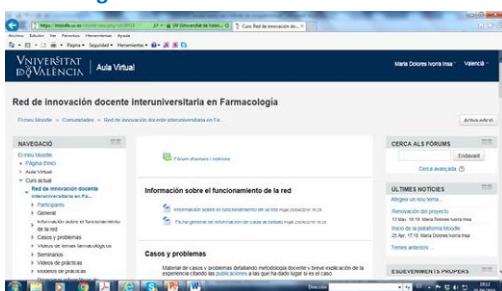
Figura 1: Plataforma Moodle
