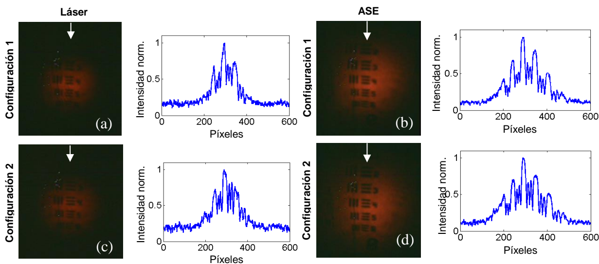
Fig. 4: Efecto del tamaño del haz ( \omega_L ) a 1064 nm en la resolución de la imagen convertida en función de la fuente de iluminación. Imagen convertida e intensidad normalizada para el corte transversal señalado ( \rightarrow ) para los casos: a) iluminación láser y \omega_L=300 \mu\text{m} , b) iluminación ASE y \omega_L=300 \mu\text{m} , c) iluminación láser y \omega_L=440 \mu\text{m} , y d) iluminación ASE y \omega_L=440 \mu\text{m} .
