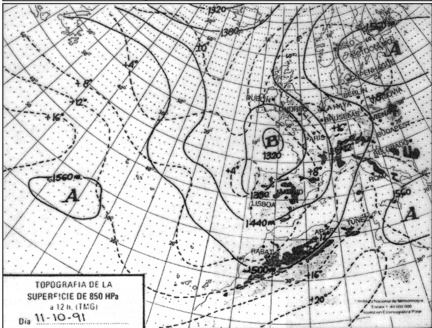
FIGURA 7. Situación correspondiente al día 11 de octubre de 1991. Las precipitaciones de polvo desértico fueron abundantes sobre las Islas Británicas. La imagen refleja la gran escala del movimiento de transporte.
