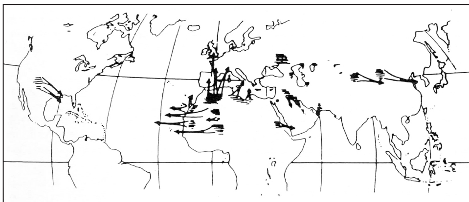
FIGURA 3. Áreas planetarias fuente de polvo atmosférico y trayectorias más frecuentes. (GRIGORYEV, A. A., y KONDRATYEV, K. J. 1980; modif. QUEREDA, J. y OLCINA, J. 1993).
