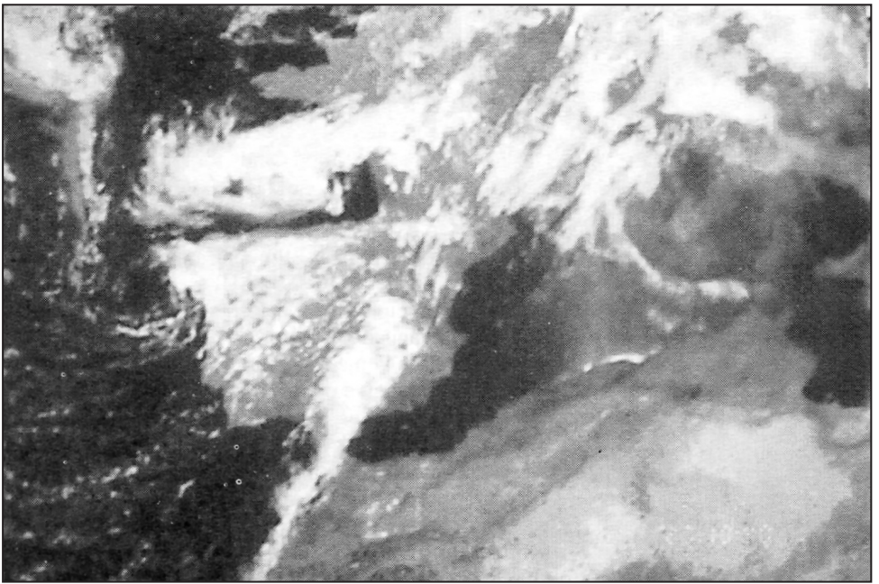
FIGURA 5. La imagen muestra la evidente coincidencia de contornos, sobre el centro de la Cuenca Occidental del Mediterráneo, entre la nube de polvo sahariano y la advección de masa aérea africana plasmada en la topografía de 850 hPa. (I.N.M. e imagen NOAA, Estación de Climatología, Universidad Jaume I, Castellón, 27 de mayo de 1993).
