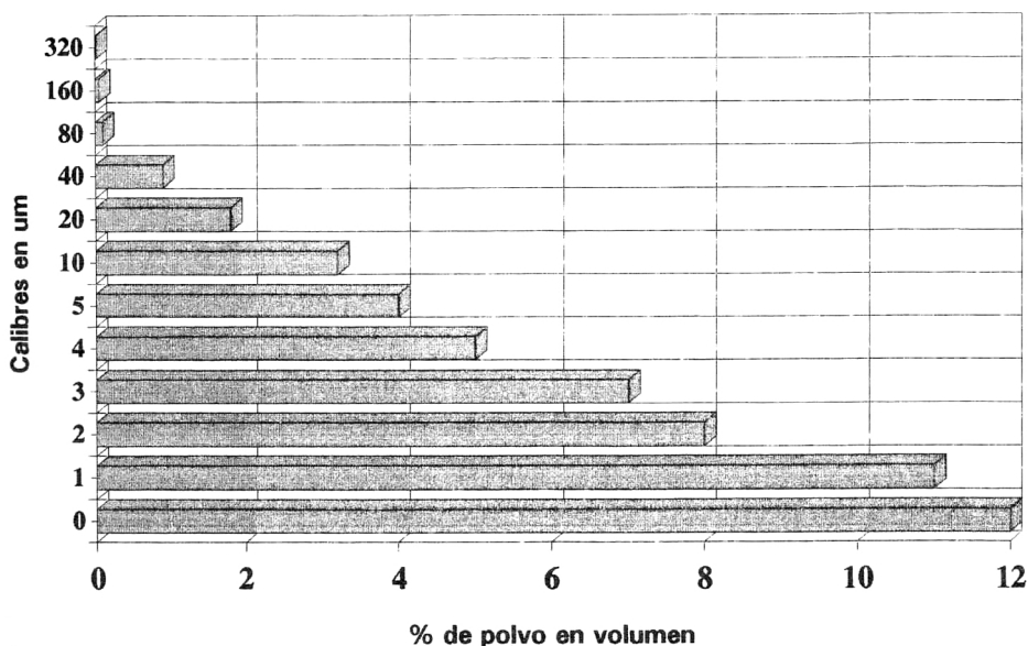
FIGURA 2. Histograma granulométrico correspondiente al episodio de lluvia de tierra del 19 de septiembre de 1993. Instituto Universitario de Tecnología Cerámica, Universidad Jaime I de Castellón.
