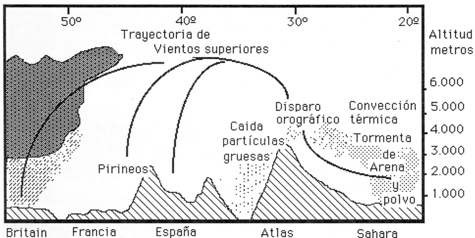
FIGURA 4. La principal fuente de polvo atmosférico para Europa es el desierto de Sahara. Una de las trayectorias más características, con toda su complejidad, es la representada en la figura.
