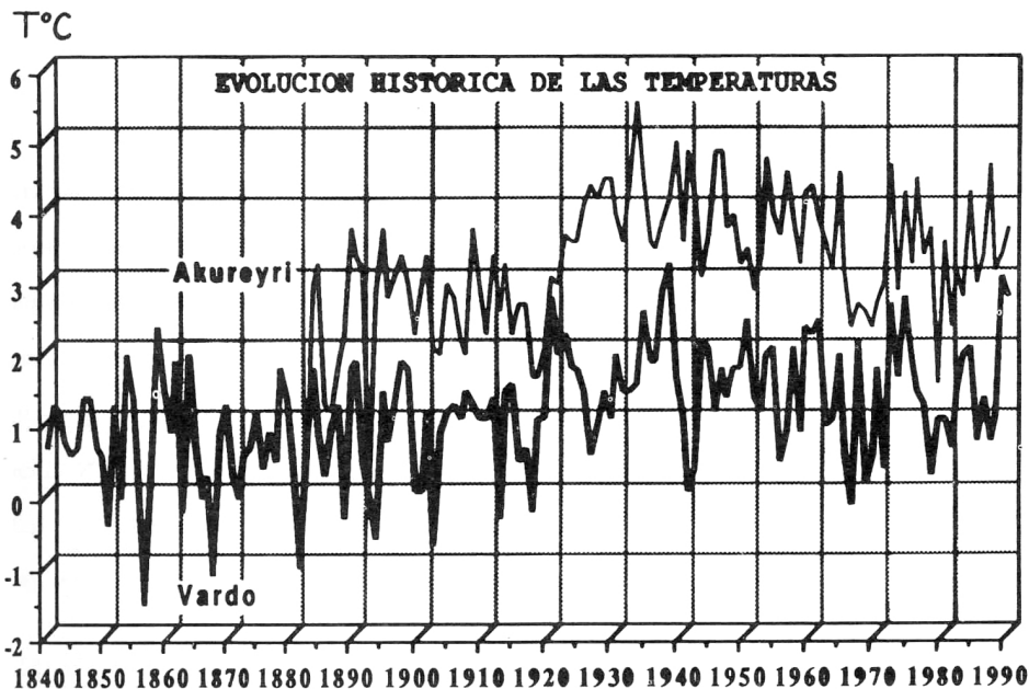
FIGURA 10. Las series térmicas de los observatorios más septentrionales del Hemisferio Norte muestran la elevación de temperaturas que se viene registrando a lo largo del siglo XX.
