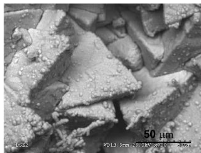
Fig. 5.- Fotomicrografía de MEB en modo de electrones retrodispersados mostrando cristales de calcita recubiertos por oxihidróxidos de hierro. Fig. 5.- SEM-bse microphotographs of calcite crystals recovered by Fe-oxyhydroxides.
