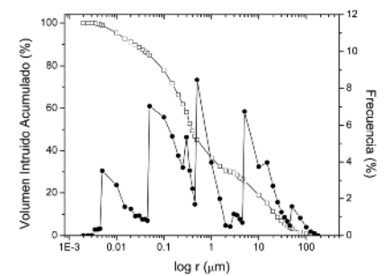
Fig. 7.- Distribución del tamaño de poro de una muestra característica del travertino del Cerro de La Almagra. Fig. 7.- Pore size distributions of a representative sample of Cerro de La Almagra travertine.
