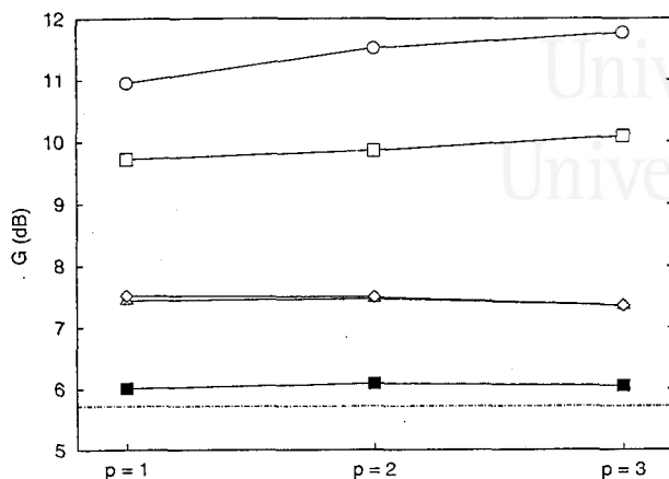
Figura 9.2: Ganancias de predicción para la señal 1 con la RRS y DG (□), FKED (○), DG+LMS (△), FKED+LMS (◇) y FKED+RLS (■). La línea constante representa el rendimiento base, \hat{u}[t+1] = u[t] .
