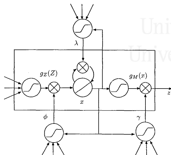
Figura 3.8: Un bloque de memoria con conexiones de mirilla, que conectan el estado del CEC con cada una de las compuertas.
