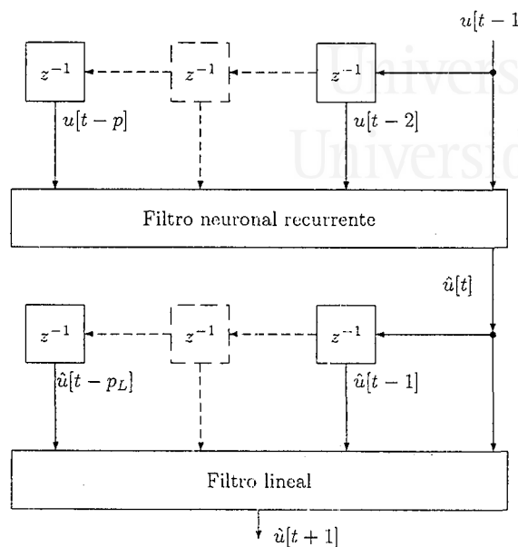
Figura 9.1: Modelo de predictor que combina filtros lineales y no lineales (Haykin y Li 1995).
