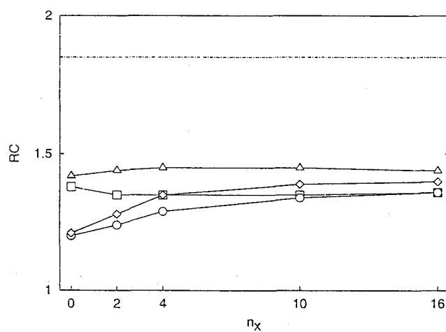
Figura 6.11: Razones de compresión para la secuencia en inglés vidwchdg. Se muestran los resultados con RPR y descenso por el gradiente ( \square ), RRS y descenso por el gradiente ( \nabla ), RPR y FKED ( \Delta ), y RRS y FKED ( \diamond ). La línea constante es la razón de compresión del modelo de [0,4] -gramas, indicada también en el cuadro 6.2.
