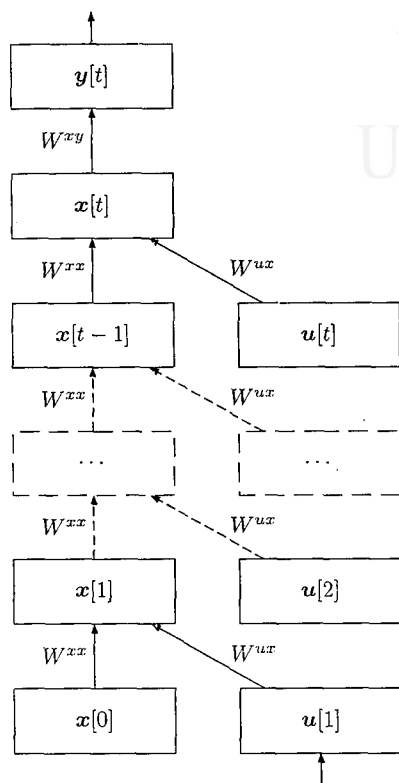
Figura 4.1: Una RRS desplegada en el instante t según BPTT.
