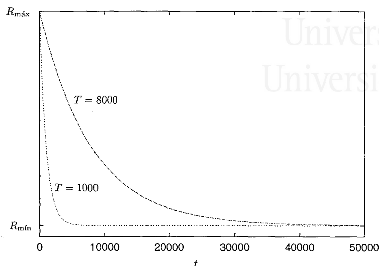
Figura 4.2: Evolución de la matriz de covarianza del error del FKED según la tasa T .
