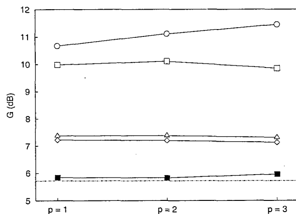
Figura 9.3: Ganancias de predicción para la señal 1 con RPR y DG (□), FKED (○), DG+LMS (△), FKED+LMS (◇) y FKED+RLS (■). La línea constante representa el rendimiento base, \hat{u}[t+1] = u[t] .
