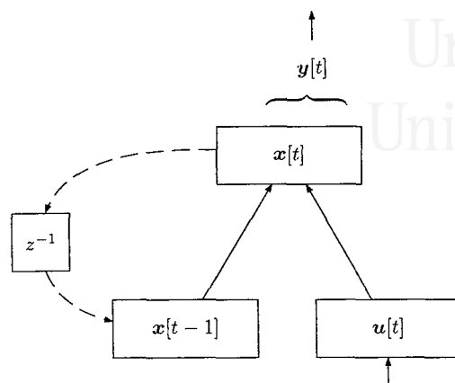
Figura 3.3: Esquema de la red totalmente recurrente de primer orden (Williams y Zipser 1989).
