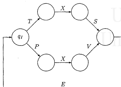
Figura 6.1: Diagrama de transiciones de la FSEF 1. El símbolo inicial aparece etiquetado como q_I . Todas las transiciones que parten de un mismo estado son equiprobables.
