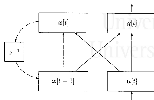
Figura 3.1: Esquema de la red parcialmente recurrente de primer orden (Robinson y Fallside 1991). El bloque etiquetado con z^{-1} representa un vector de células de retardo temporal.
