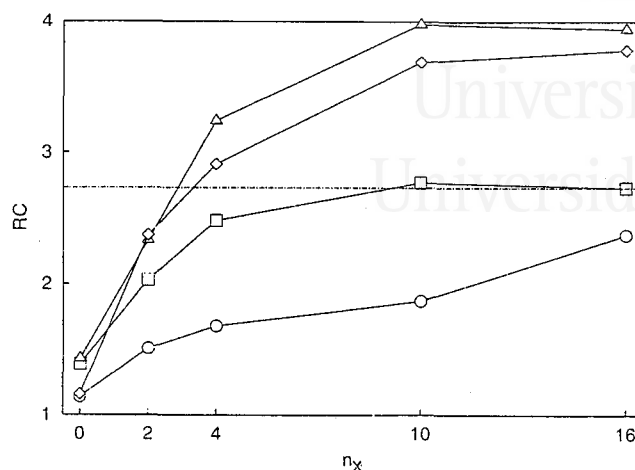
Figura 6.8: Razones de compresión para la secuencia del láser caótico. Se muestran los resultados con RPR y descenso por el gradiente ( \square ), RRS y descenso por el gradiente ( \circ ), RPR y FKED ( \triangle ), y RRS y FKED ( \diamond ). La línea constante es la razón de compresión del modelo de [0, 4] -gramas.
