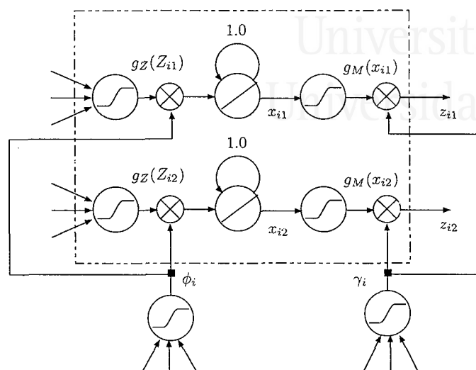
Figura 3.5: El bloque de memoria i -ésimo con dos celdas.
