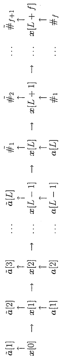
Figura 8.1: Primera fase del entrenamiento: predicción de la siguiente clase de ambigüedad. el símbolo “ \tilde{\cdot} ” significa valor predicho ; los “ \# ” son los marcadores de final de frase. Nótese la secuencia de f marcadores de final de frase, necesaria para poder etiquetar las últimas f palabras de cada frase en la segunda fase del entrenamiento.
