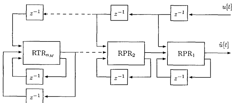
Figura 3.9: Esquema de la red recurrente en cascada (Haykin y Li 1995).
