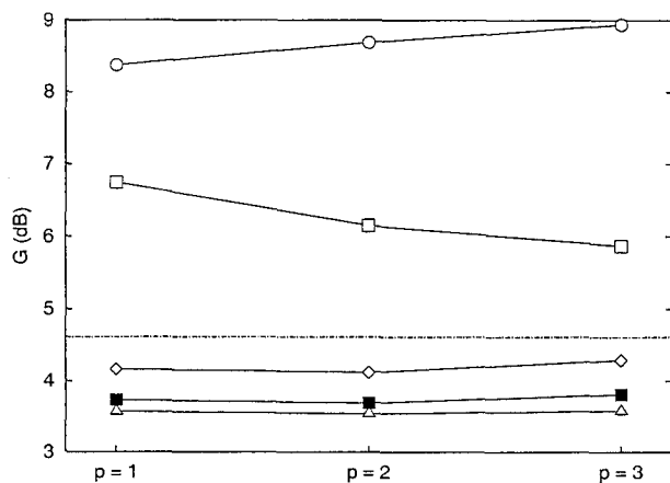
Figura 9.6: Ganancias de predicción para la señal 3 con RRS y DG (□), FKED (○), DG+LMS (△), FKED+LMS (◇) y FKED+RLS (■). La línea constante representa el rendimiento base, \hat{u}[t+1] = u[t] .
