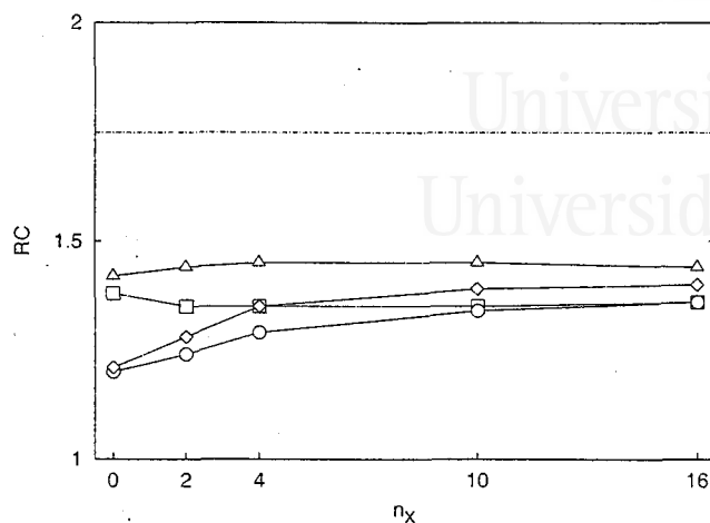
Figura 6.10: Razones de compresión para la secuencia en inglés kiesdis3. Se muestran los resultados con RPR y descenso por el gradiente ( \square ), RRS y descenso por el gradiente ( \nabla ), RPR y FKED ( \Delta ), y RRS y FKED ( \diamond ). La línea constante es la razón de compresión del modelo de [0,4] -gramas, indicada también en el cuadro 6.2.
