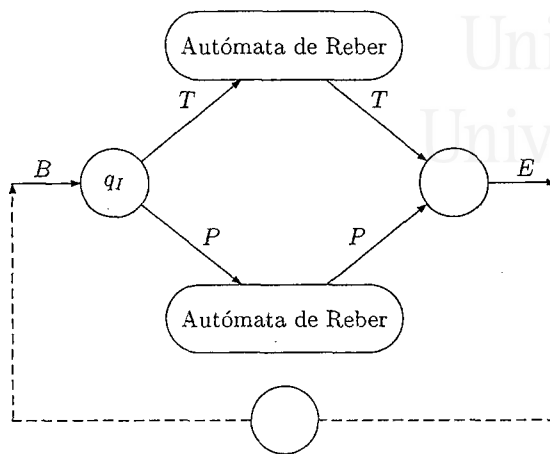
Figura 6.4: Diagramas de transiciones para la FSEF 3, obtenida a partir del autómata de Reber de la figura 6.3. Todas las transiciones que parten de un mismo estado son equiprobables. Las transiciones no mostradas en el diagrama tienen probabilidad nula. La línea inferior indica la variante continua; la discontinua se conoce normalmente como autómata de Reber simétrico.
