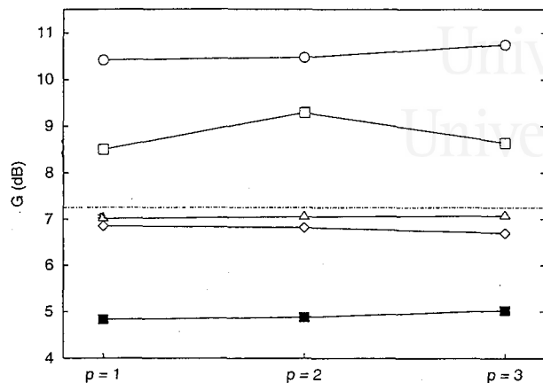
Figura 9.5: Ganancias de predicción para la señal 2 con RPR y DG (□), FKED (○), DG+LMS (△), FKED+LMS (◇) y FKED+RLS (■). La línea constante representa el rendimiento base, \hat{u}[t+1] = u[t] .
