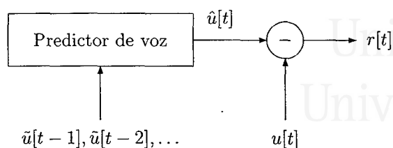
Figura 1.1: Esquema de la codificación predictiva sobre una señal u[t] . La señal enviada por el canal (después de ser codificada) es r[t] .
