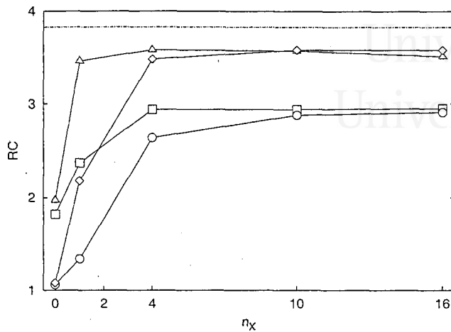
Figura 6.6: Razones de compresión para la secuencia derivada de la FSEF 2. Se muestran los resultados con RPR y descenso por el gradiente ( \square ), RRS y descenso por el gradiente ( \circ ), RPR y FKED ( \triangle ), y RRS y FKED ( \diamond ). La línea constante es la razón de compresión del modelo de [0, 4] -gramas, indicada también en el cuadro 6.1.
