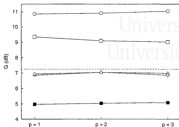
Figura 9.4: Ganancias de predicción para la señal 2 con RRS y DG (□), FKED (○), DG+LMS (△), FKED+LMS (◇) y FKED+RLS (■). La línea constante representa el rendimiento base, \hat{u}[t+1] = u[t] .
