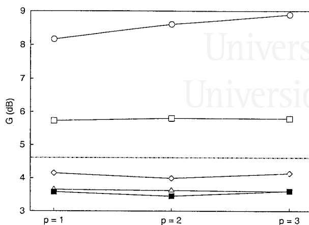
Figura 9.7: Ganancias de predicción para la señal 3 con RPR y DG (□), FKED (○), DG+LMS (△), FKED+LMS (◇) y FKED+RLS (■). La línea constante representa el rendimiento base, \hat{u}[t+1] = u[t] .
