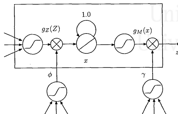
Figura 3.4: Un bloque de memoria con una única celda. La entrada de la celda se representa con Z , la activación de la compuerta de entrada con \phi , la activación de la compuerta de salida con \gamma , la activación del CEC con x y la activación global de la celda con z .
