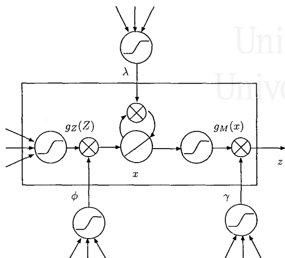
Figura 3.7: Un bloque de memoria con una compuerta de olvido con activación \lambda .
