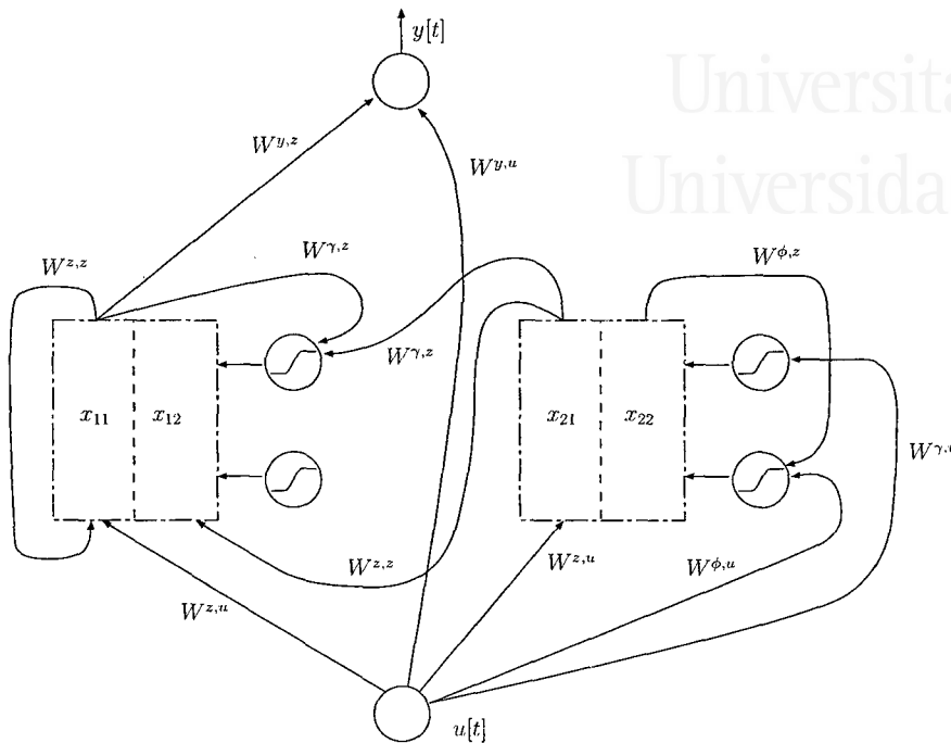
Figura 3.6: Una red LSTM con dos bloques de memoria de dos celdas cada uno. Solo se muestran algunas conexiones y no se muestran los sesgos.
