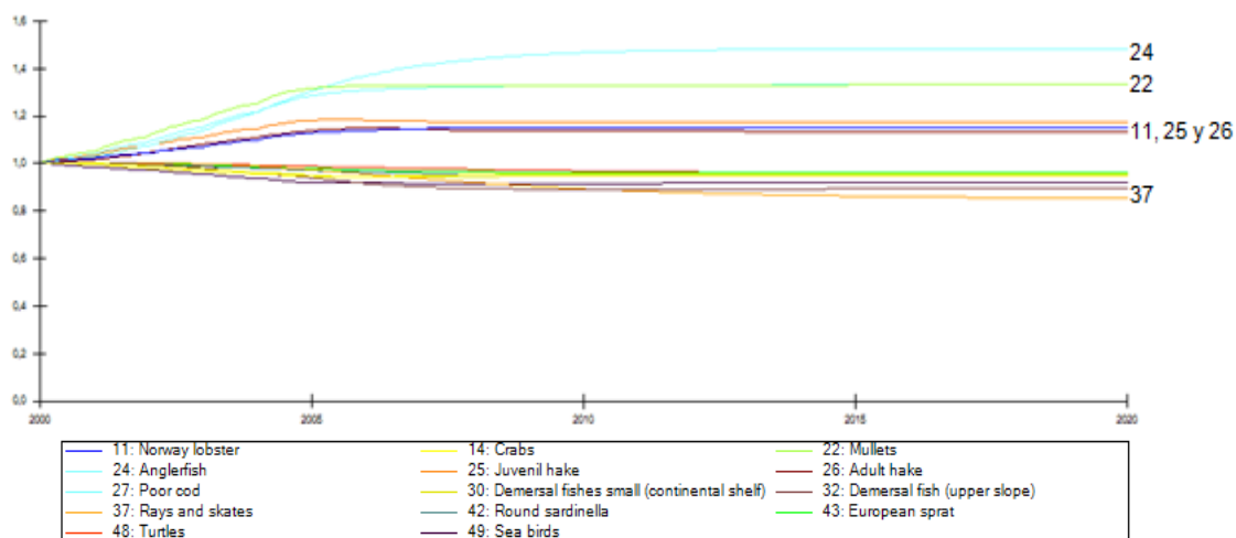
Figura 13. Resultados de la simulación de reducción de un 20% del esfuerzo pesquero de la flota de arrastre. En esta figura solo se muestran los grupos funcionales con una variación de su biomasa destacable (mayor al 10%).
