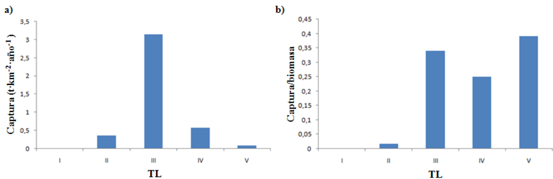
Figura 12. Captura (t·km 2 ·año -1 ) y cociente captura/biomasa por nivel trófico entero.
