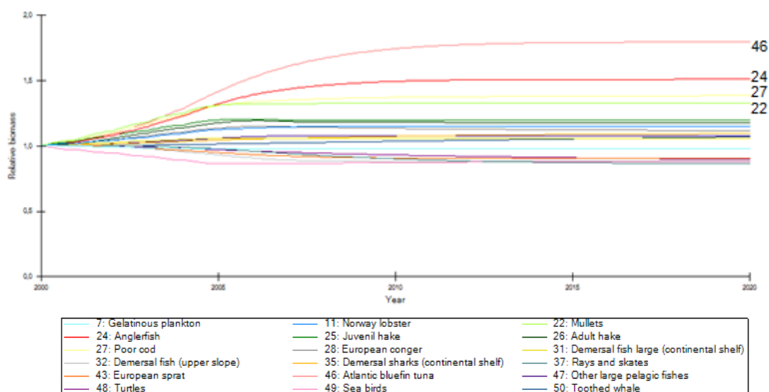
Figura 16. Resultados de la simulación preliminar de reducción de un 20% del esfuerzo pesquero de las flotas de arrastre, cerco y palangre. En esta figura solo se muestran los grupos funcionales que muestran una variación de su biomasa destacable
