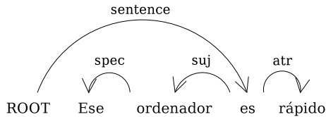
Figura 1: Ejemplo de árbol de dependencias
