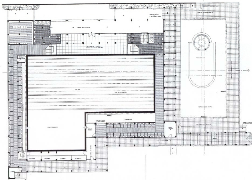
Balneario Las Arenas 1933-34, Piscinas, Gutiérrez Soto
