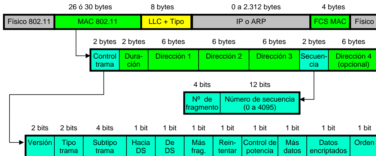
Figura 11. Formato de una trama IEEE 802.11 con un paquete IP o ARP.
