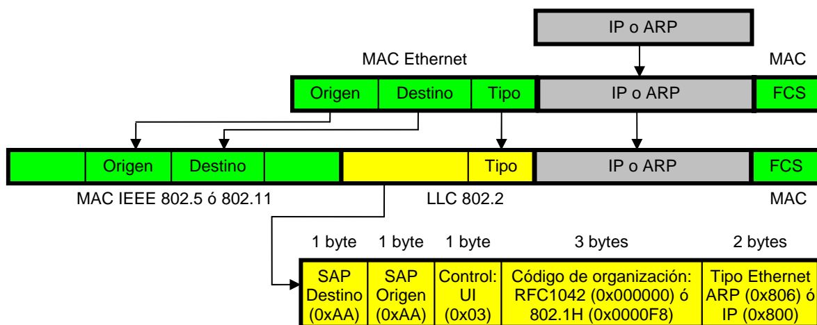
Figura 10. Encapsulación Ethernet: paquetes IP o ARP sobre otras LAN.
